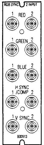
Figure 2-16. RGB Sync 2 Input Module
